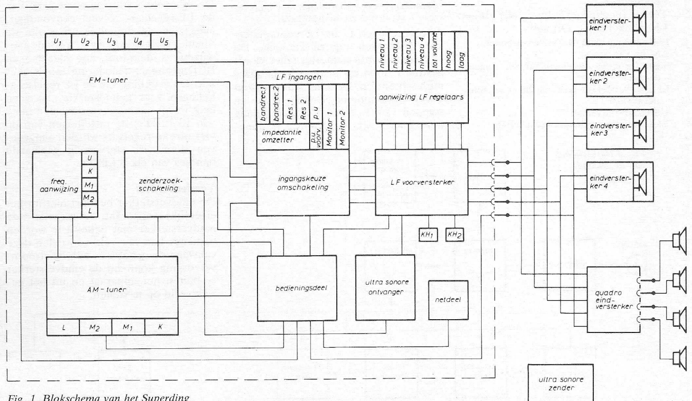
Fig. 1. Blokschema van het Superding
