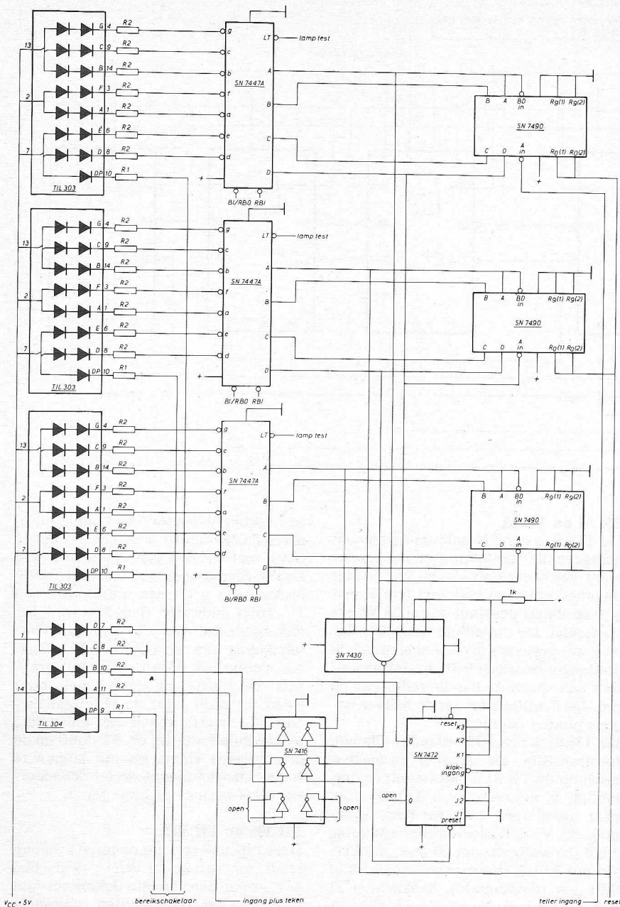
Fig. 3. Een 3 1 / 2 cijfer indicator.
