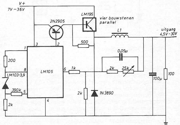
Fig. 3. Volledig schema van de interne schakeling.
