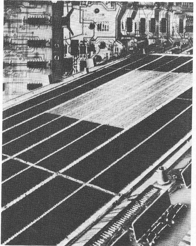
Het nieuwe, voor Digital's PDP-11 minicomputers ontworpen, high-speed 16 k computergeheugen.
