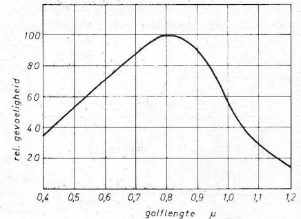
Fig. 2. Gevoeligheidskromme.
