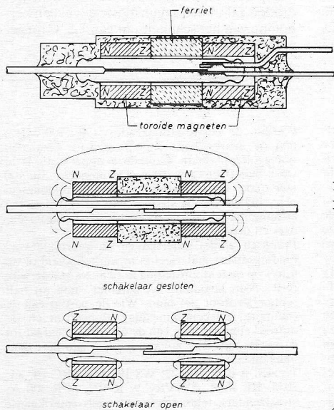
Fig. 1 tm 3 (boven): Verschillende uitvoeringsvormen van temperatuurgevoelige reed-relais.
