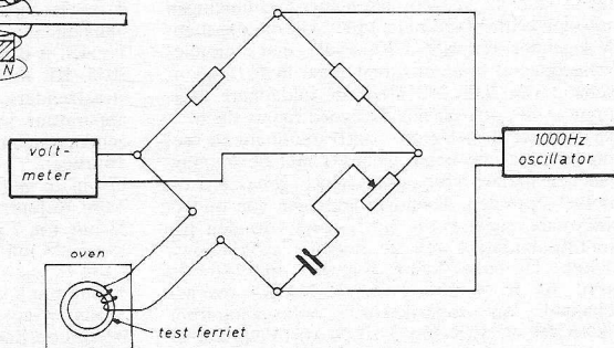
Fig. 5. Testschakeling
